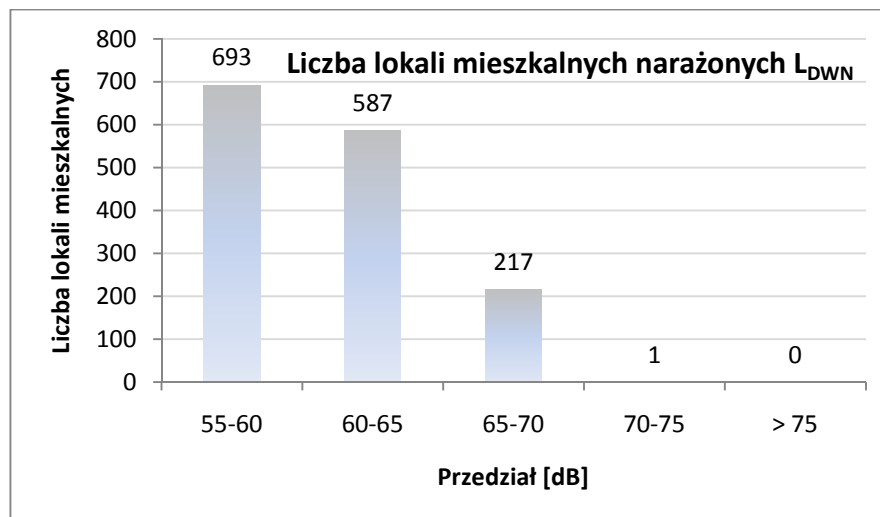
Rys. 4.3 Liczba lokali mieszkalnych narażonych na hałas wyrażony wskaźnikiem L_{DWN}
